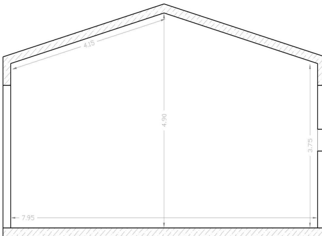
Τομή A-A'
